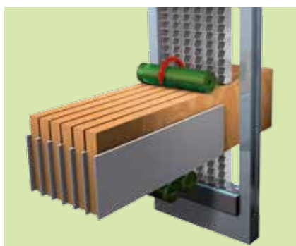
6-kanałowy kanał podawczy
