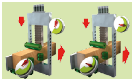
Sterowany elektronicznie precyzyjny posuw
