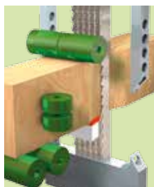
Układ stabilizacji
